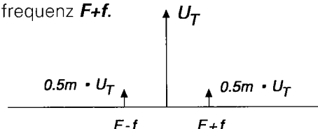
Figur 1 Spektrumsamplituden und -frequenzen bei AM (m = 50%)
